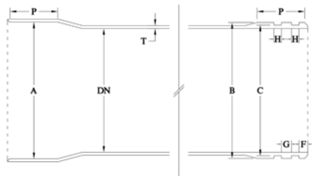
Dimensiones típicas para tubería con PN 10
