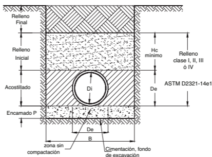
Figura 3. Sección de zanja típica para tubería de polietileno y polipropileno, conforme a norma ASTM D2321-14e1.
