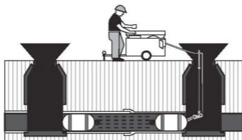
Figura 31. Colocación de tapones inflables para prueba de hermeticidad de campo.
